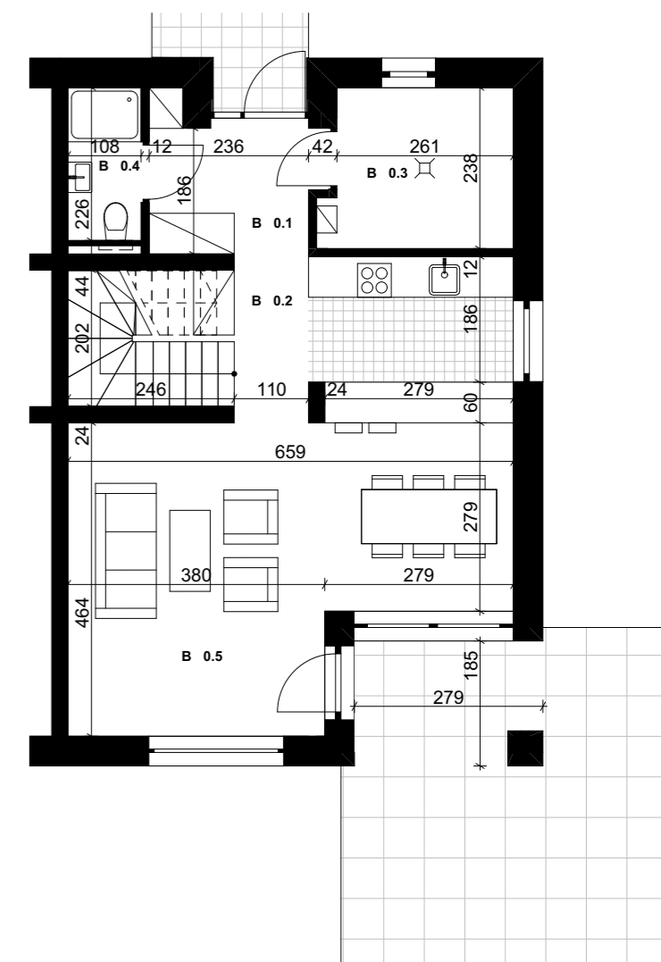
Rzut parteru
